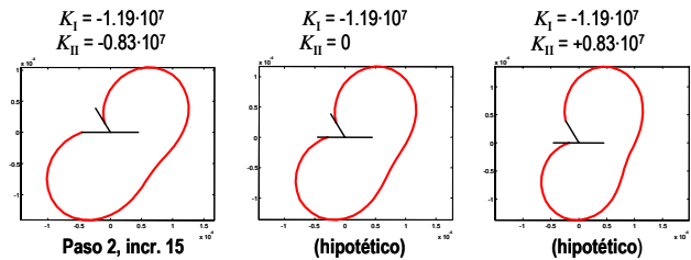
Fig. 12. Variación del isocontorno de von Mises (paso 2, incr. 15) suponiendo valores hipotéticos de K_{II} .
