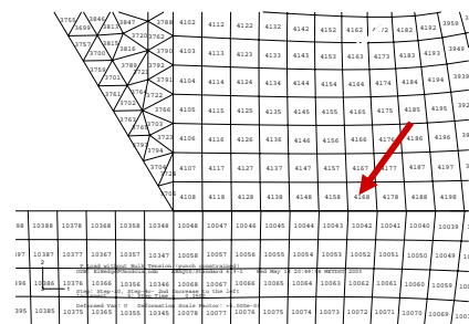
Fig. 10. Elemento junto al plano de contacto para el que se estudia la transición adhesión-deslizamiento.
