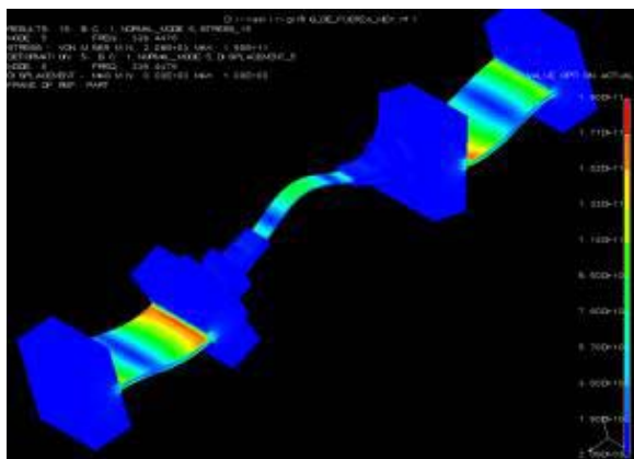
Fig 2. Uno de los modos normales de vibración del sistema de ensayo. Un modelo más completo que el representado es necesario para un correcto diseño.
