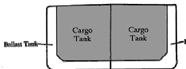
Fig. 7 – Esquema doble casco
