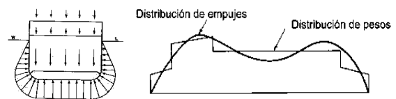
Fig. 4 – Cargas transversales y longitudinales
